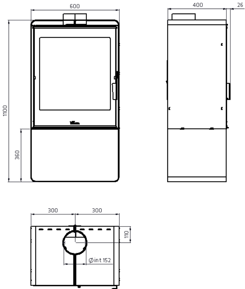
Figura nº1 - Dimensiones en mm de la serie Ocean/Atlantic 610
