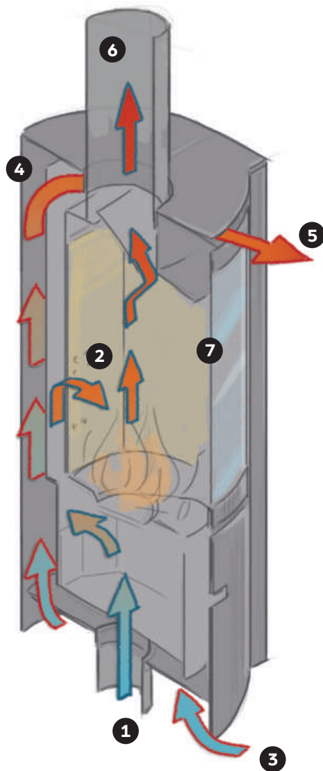
Técnica de combustión y circulación del aire Ståv 30-compact
