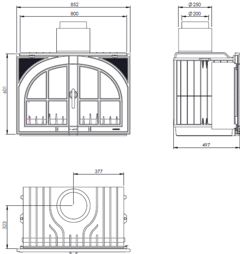
Figura n°1 - Dimensiones en mm del aparato Sara
