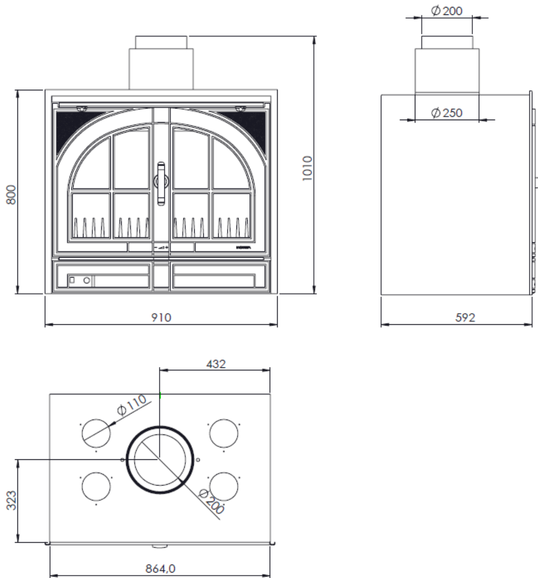
Figura n°2 - Dimensiones en mm del aparato Abodi
