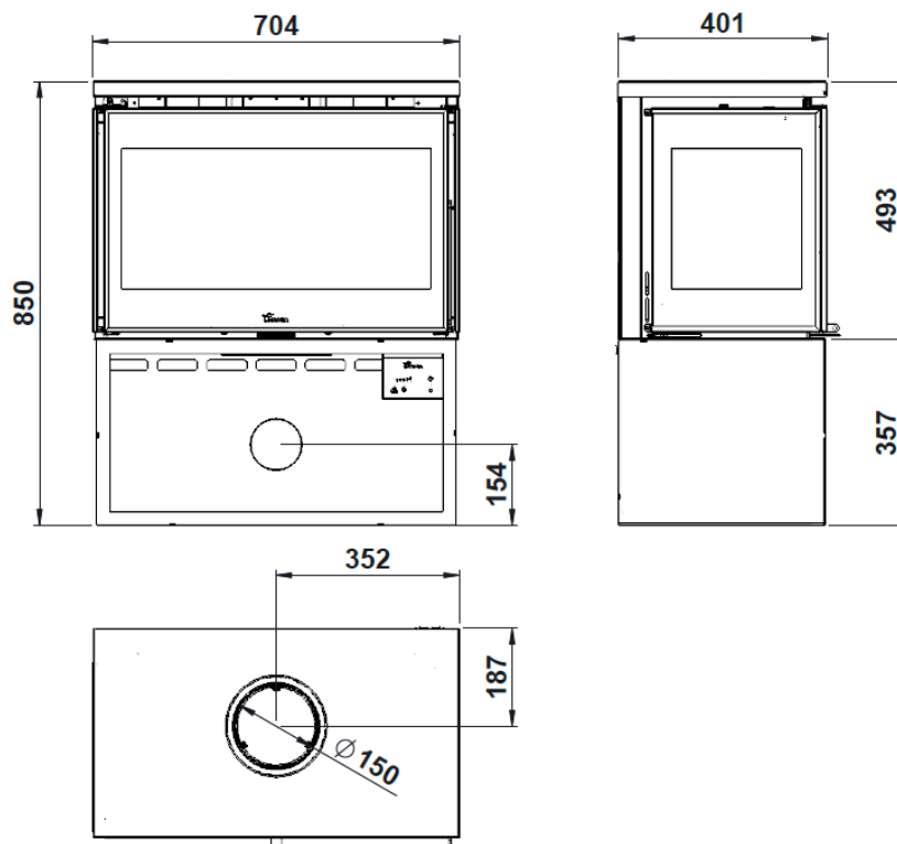
Figura n°2 - Dimensiones en mm del aparato PARIS 700 CLID
